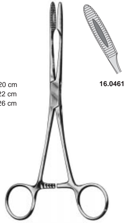
MAIER 16.0460 25 cm
